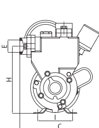
Габаритные и присоединительные размеры AUPS 126
