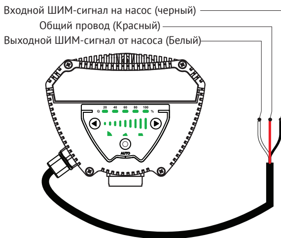
Рисунок 11 – Кабель ШИМ-сигнала
