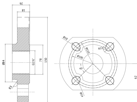
Размеры фланца из комплекта поставки
