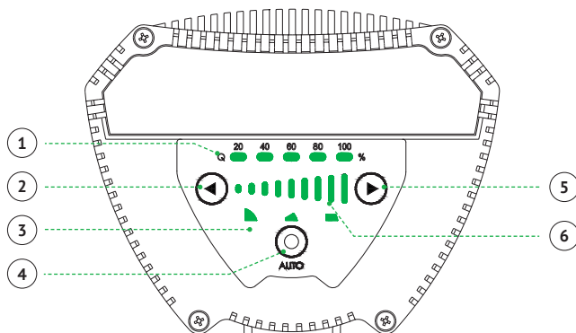
Рисунок 3 – Панель управления
